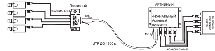
2) Пассивно-активная передача видеосигнала
