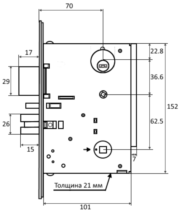
Электромеханический замок
