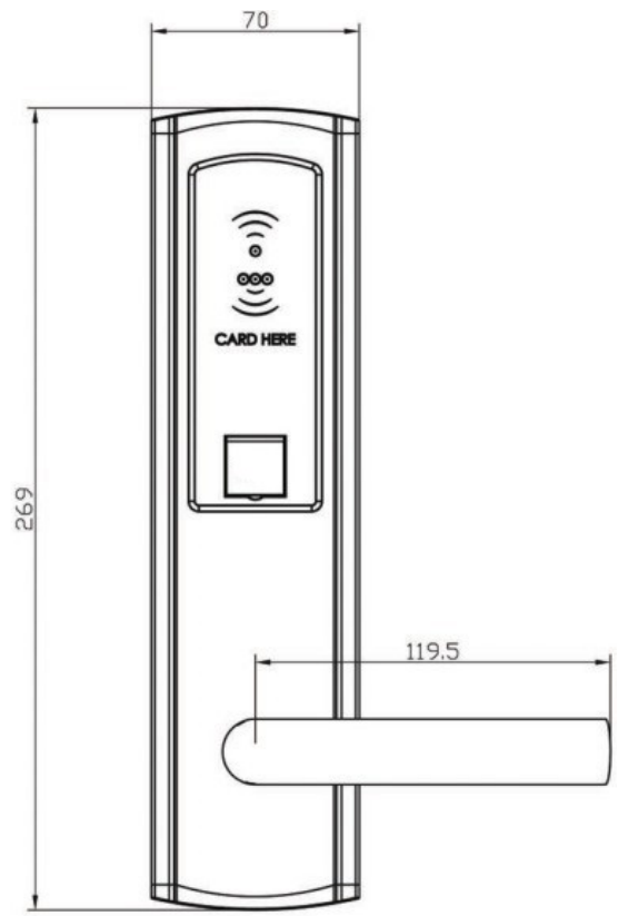
Внешняя ручка-накладка
