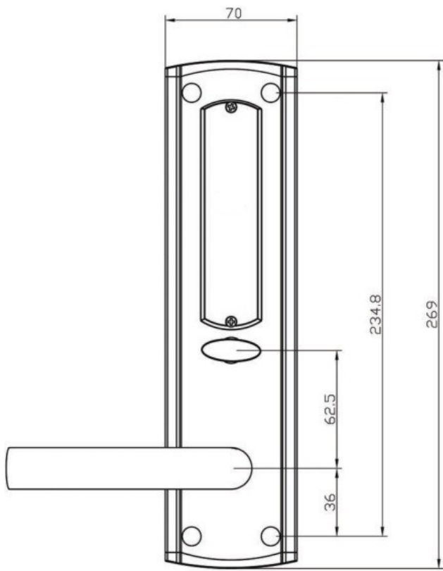
Внутренняя ручка-накладка
